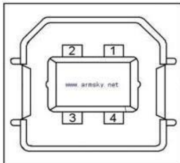
Рисунок 22. Разъем интерфейса USB
