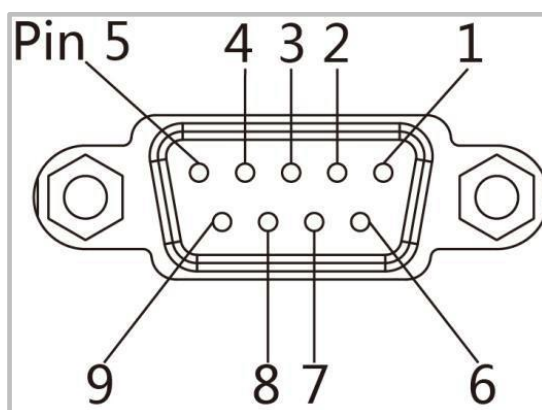
Рисунок 23. Разъем интерфейса
