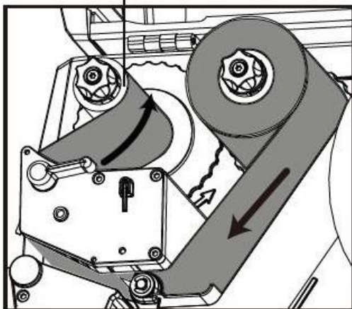
Рисунок 8. Схема загрузки красящей ленты
